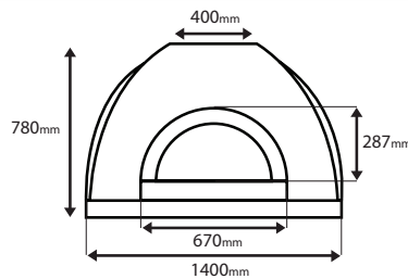
Oven Diagram (voorkant)
